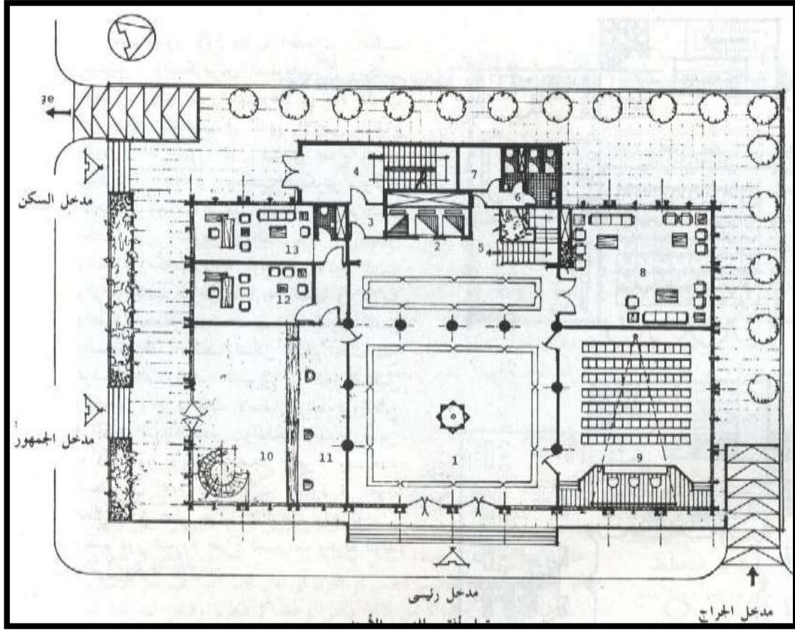
الشكل (4-8): الطابق الأرضي للسفارة المصدر: (عالم البناء 91، 1988)
