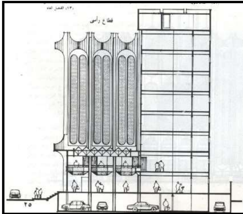
الشكل (4-12): مقطع طولي للسفارة المصدر: (عالم البناء 91، 1988)
