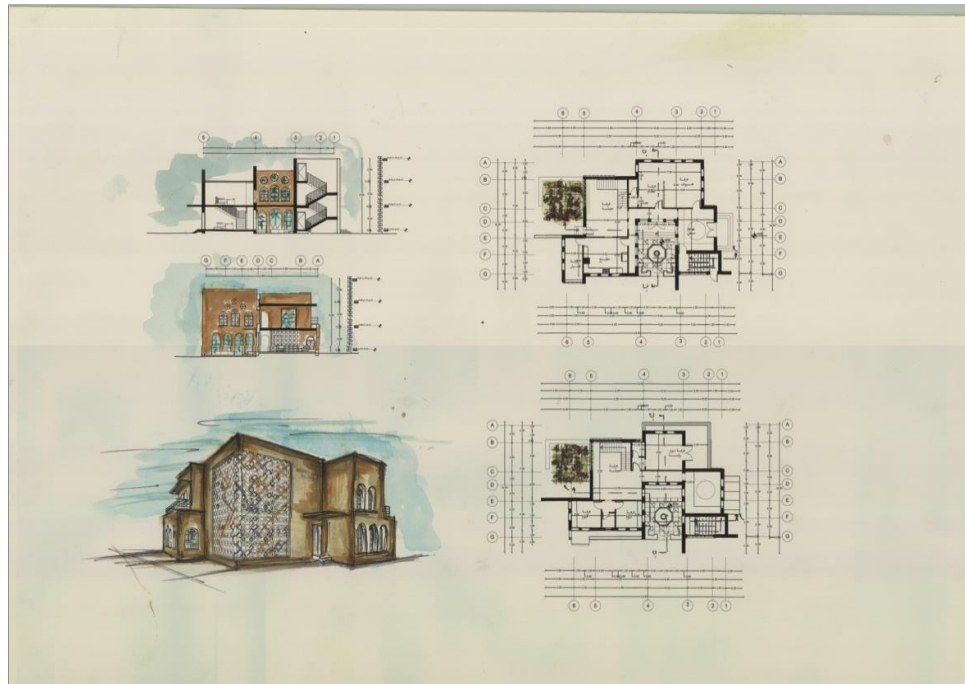
الصورة 14.8 (المساقط الافقية مع الأبعاد والمقاطع)
