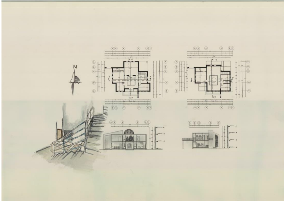
الصورة 11.8 (المساقط الأفقية مع الأبعاد والمقاطع)
