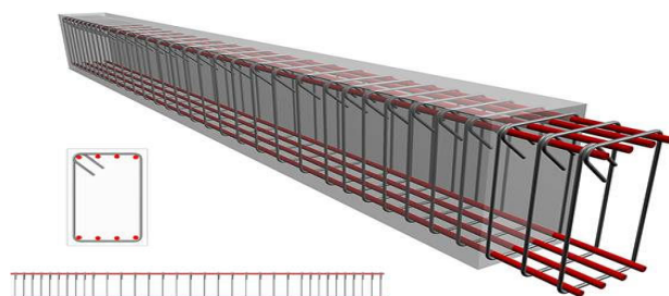
الشكل (12-3) التسليح في الجسور.
