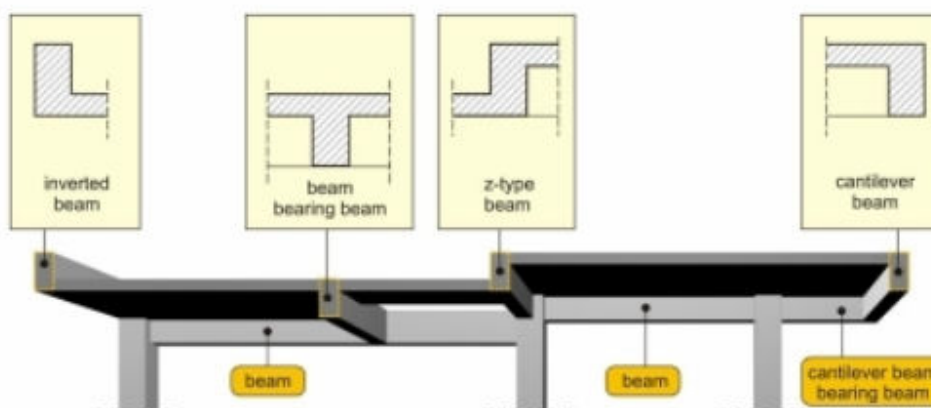
الشكل (11-3) المقاطع المختلفة للجسور في العقدات .
