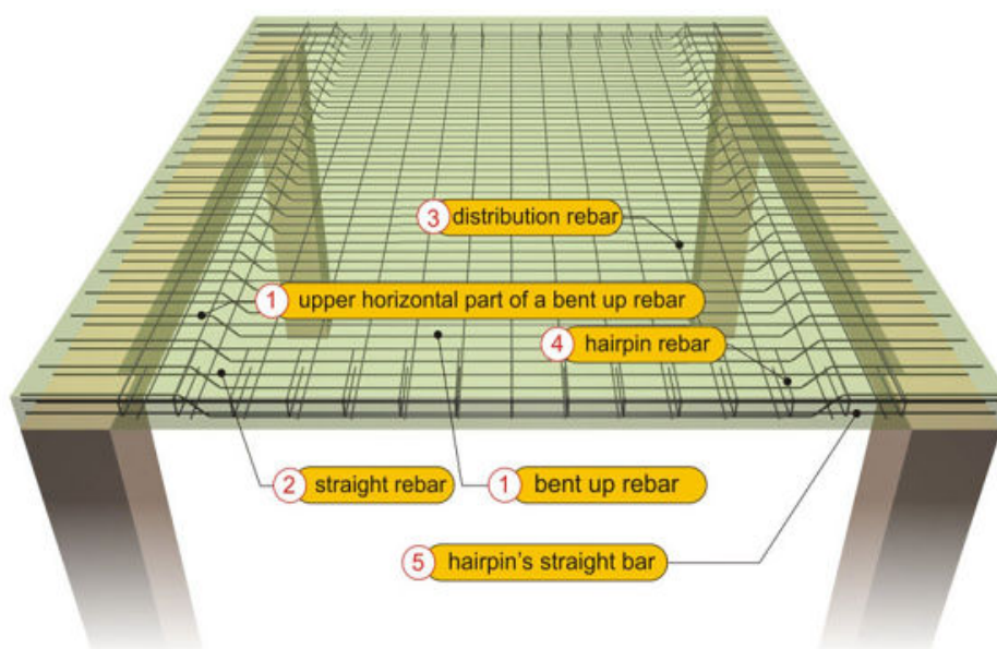
الشكل (8-3) : العقدات المصممة ذات الإتجاه الواحد One way solid slab.
