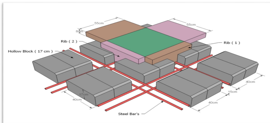
الشكل (7-3) : عقدات العصب ذات الإتجاهين.
