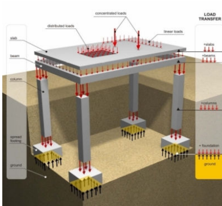
الشكل (1-3) : مسار نقل الأحمال Load path from structure to the ground
