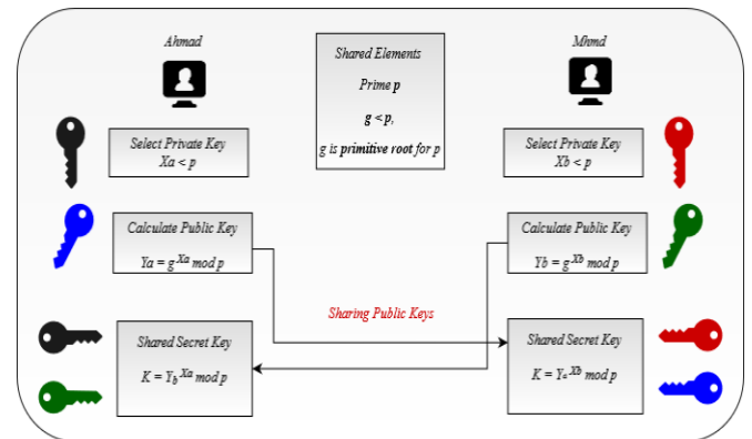
Figure 7. DH Key [21].
