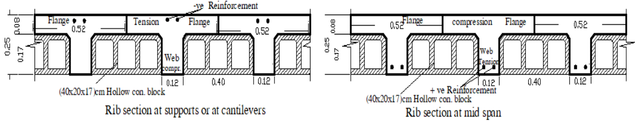
شكل 2. يبين أماكن الشد والضغط في الأعصاب باختلاف مكان المقطع
