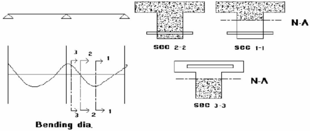
شكل 7. علاقة محور الحياد (Neutral Axis) مع مكان المقطع في العصب (المصدر: الهندي، محمد. ص 19)
