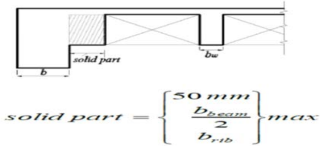
شكل 9. يوضح فكرة الجزء المصمت عند اتصال بلاطة الأعصاب مع الجسور المحيطة (المصدر: الهندي، محمد. ص 130)
