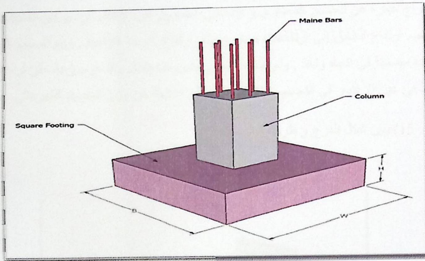
الشكل (3-12) : شكل الأساس المنفرد .
