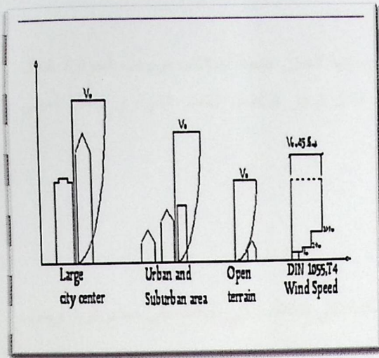
الشكل (2-3) تأثير سرعة الرياح على قيمة الضغط الواقع على المبنى
