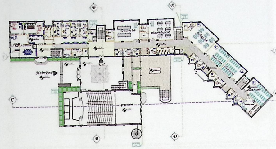
شكل (6-2) :- مخطط الطابق الأرضي.
