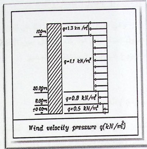
الشكل (2-3) تأثير سرعة الرياح على قيمة الضغط الواقع على المبنى
