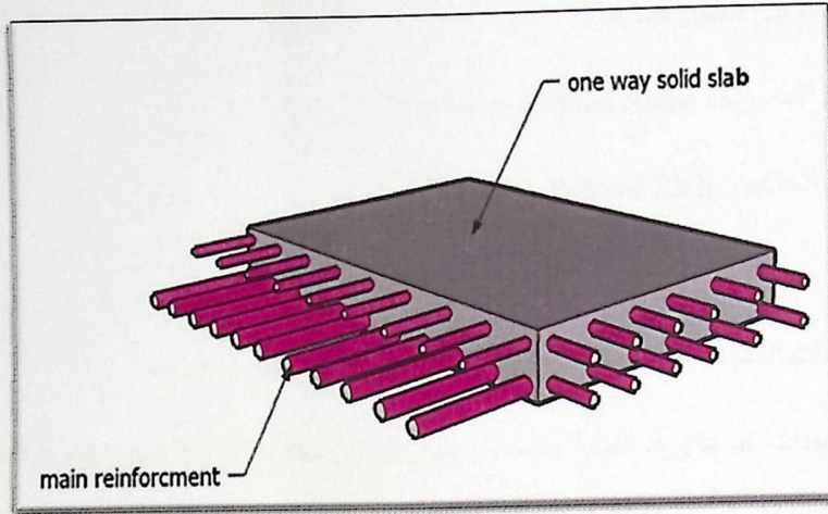
الشكل (3-5) عقدة مصمتة باتجاه واحد .
