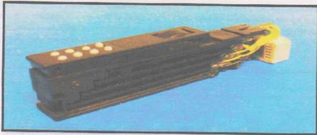
Fig. 3.10 P20 Piezoelectric Braille Cell Module
