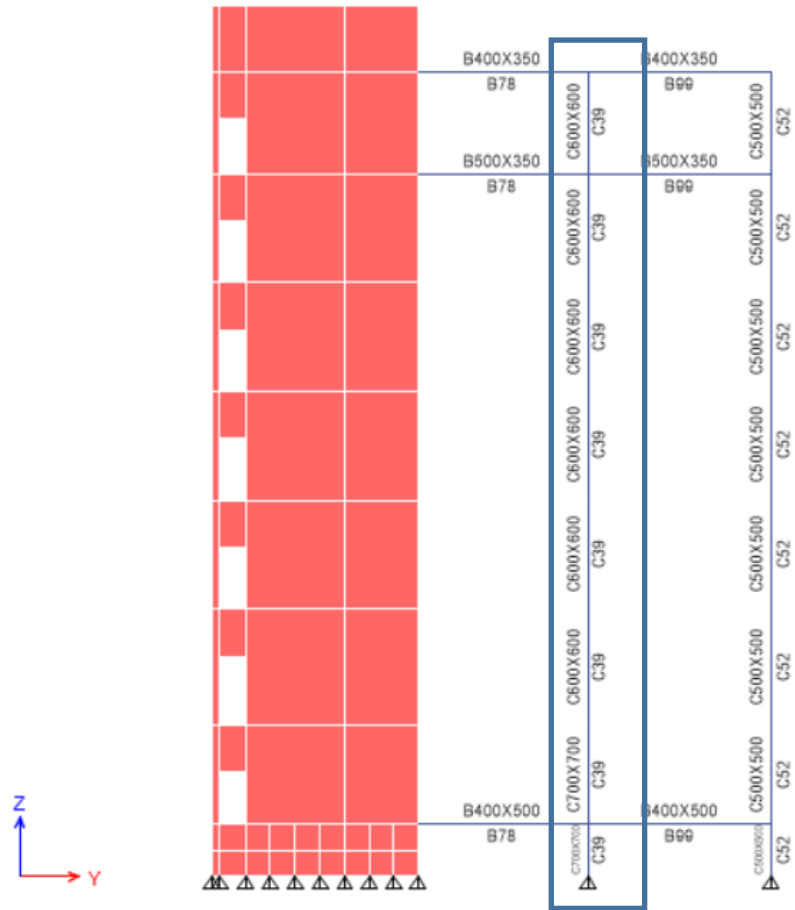
الشكل 27 Column 39 C16 Elevation
