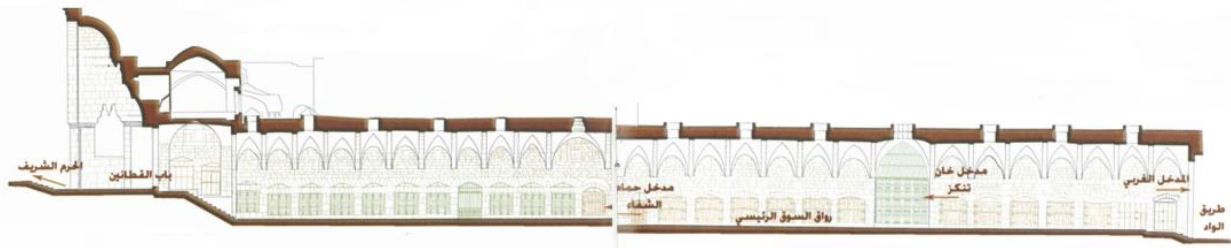
الشكل (4.5) : مقطع رأسي يمر عبر رواق السوق ويظهر به صف الدكاكين الجنوبي
