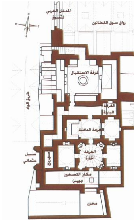
الشكل (7.5) : مسقط أفقي لحمام العين
