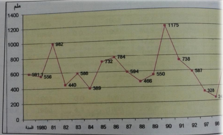
الشكل (3.6): يوضح نسبة الامطار 1998-1980 م
