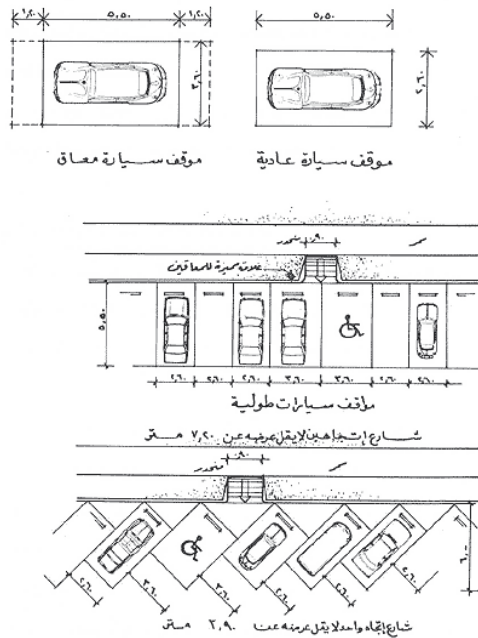
الشكل (1.4) : يوضح أنواع مواقف السيارات
