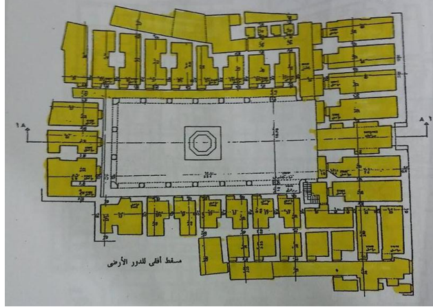
الشكل (3.1) : مسقط أفقي للدور الأرضي لوكالة الغوري
