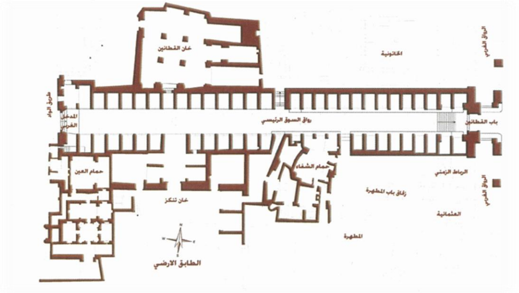
الشكل (2.5) : الطابق الأرضي لسوق القطنيين
