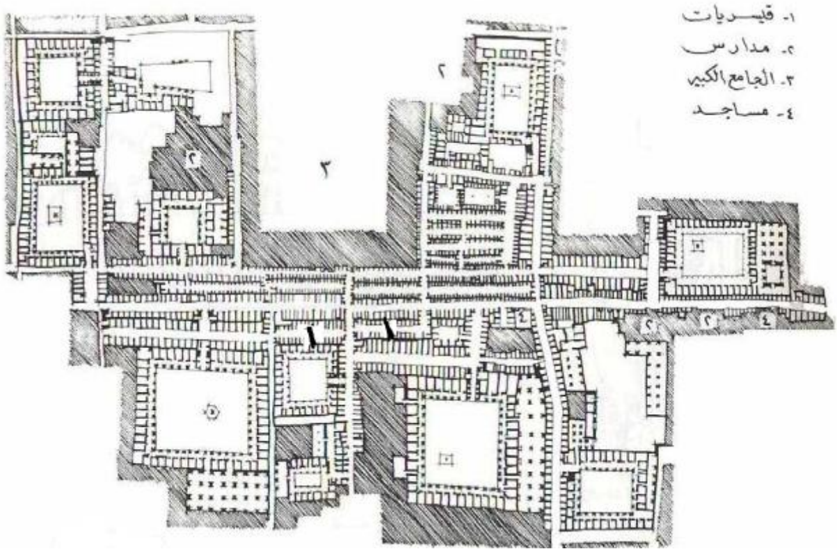
الشكل (10.2) : سوق مدينة حلب
