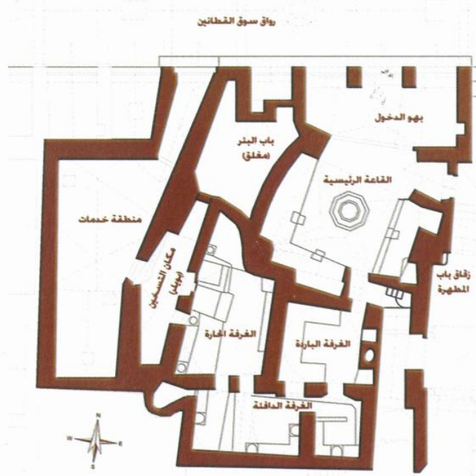
الشكل (8.5) : مسقط أفقي لحمام الشفاء
