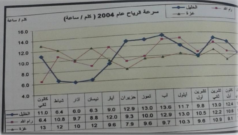
الشكل (5.6) : يوضح المعدل السنوي للرياح عام 2004
