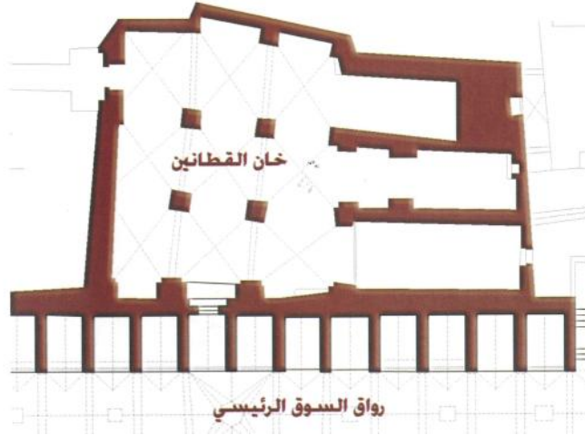
الشكل (10.5) : مسقط أفقي لخان القطنين
