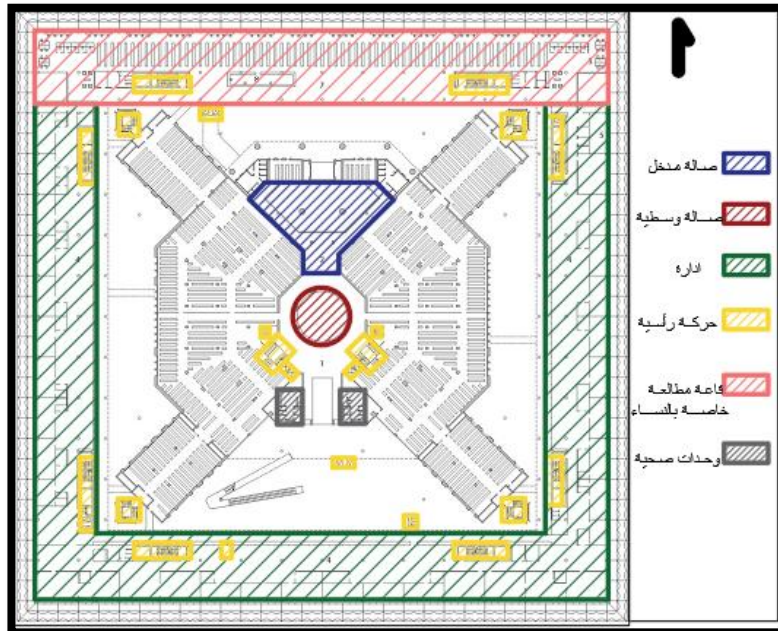
شكل (٤-٢٢): الطابق الأول
