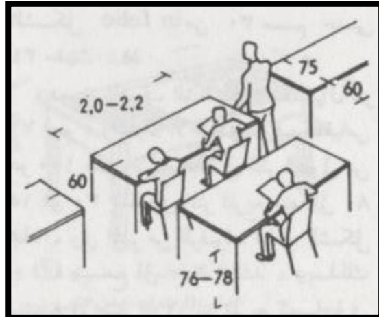
الشكل (٥-٣): طاولات طويلة المصدر: عناصر التصميم والانشاء المعماري
