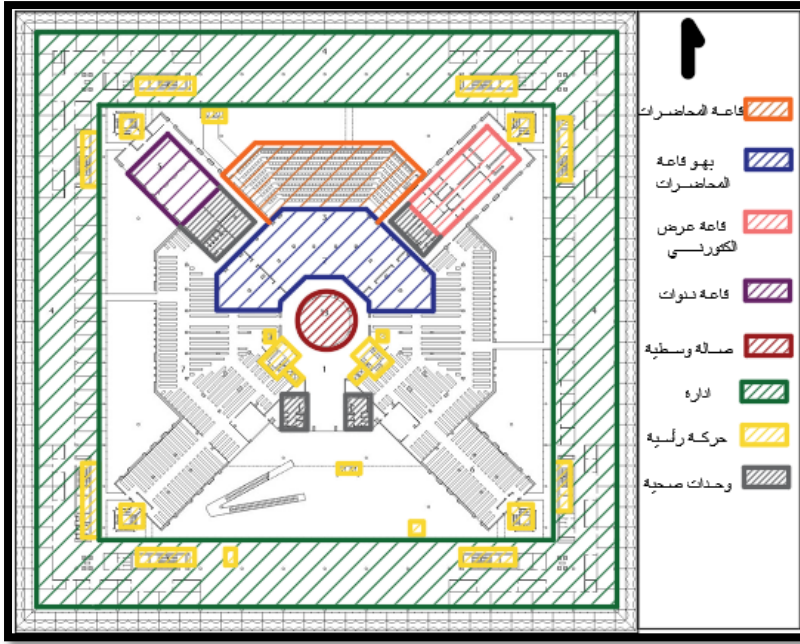
الشكل(٤-٢٣): الطابق الثاني
