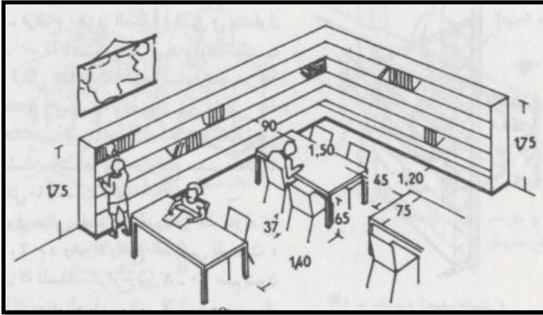
الشكل (٧-٣): قاعة مطالعة للأطفال المصدر: عناصر التصميم والانشاء المعماري
