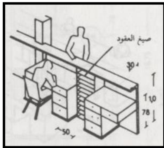
الشكل (١-٣): طاولة استعلامات للجمهور
