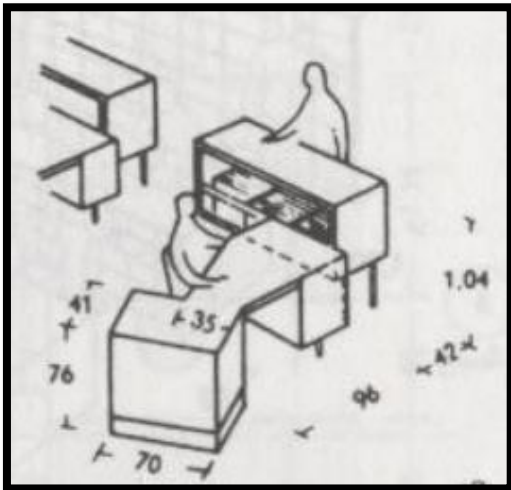
الشكل (٢-٣): شكل آخر لطاولة استعلامات للجمهور
