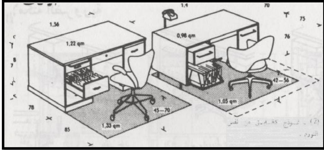
الشكل (٣-١٧): نموذج مكتب للموظفين المصدر: عناصر التصميم والانشاء
