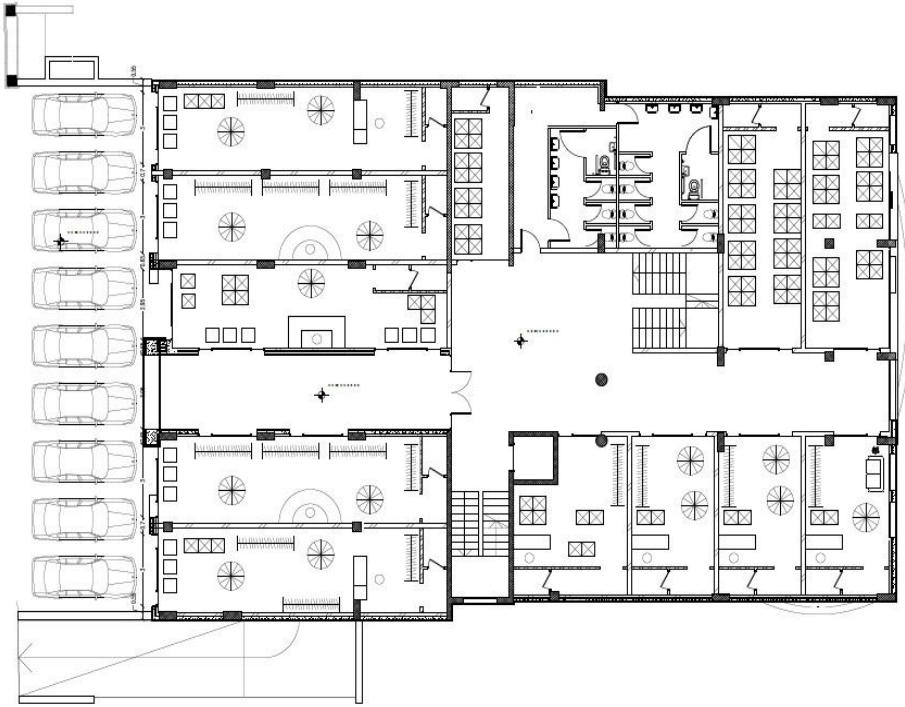
الشكل (2-5): المسقط الأفقي للطابق الارضي.
