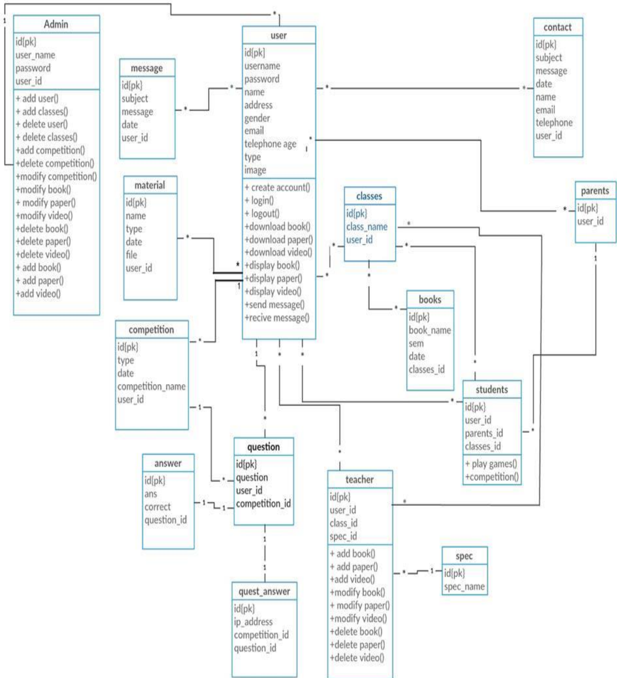
الشكل 2.6 class-diagram
